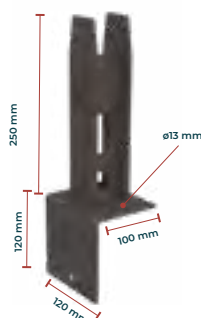
Platine à équerre pour muret 15 cm ou plus
