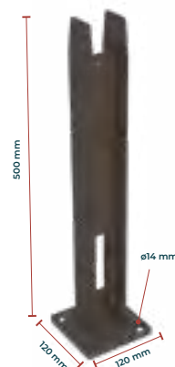
Platine renforcée pour pose d'occultant ou claustra sur muret 25 cm ou plus
